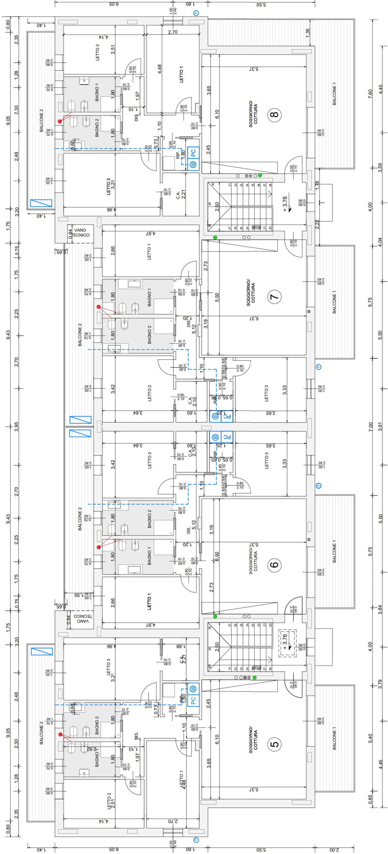
PIANTA PIANO PRIMO
