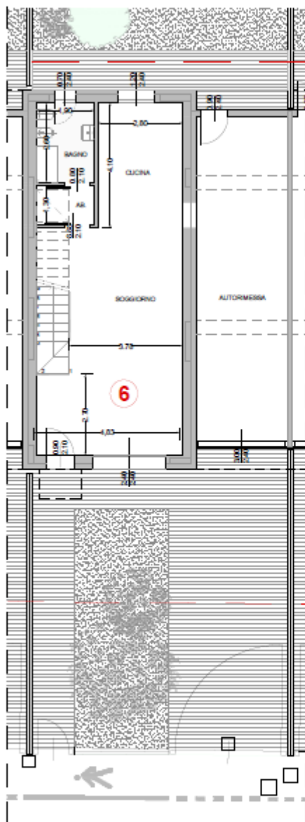
PIANTA PIANO TERRA- villa n. 6
