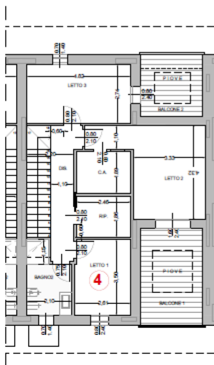
PIANTA PIANO PRIMO - villa n. 4
