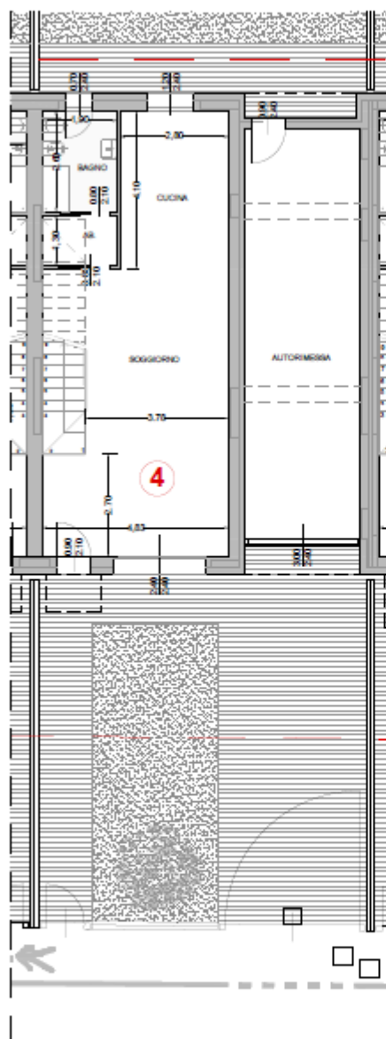
PIANTA PIANO TERRA - villa n. 4
