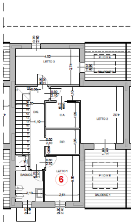
PIANTA PIANO PRIMO - villa n. 6
