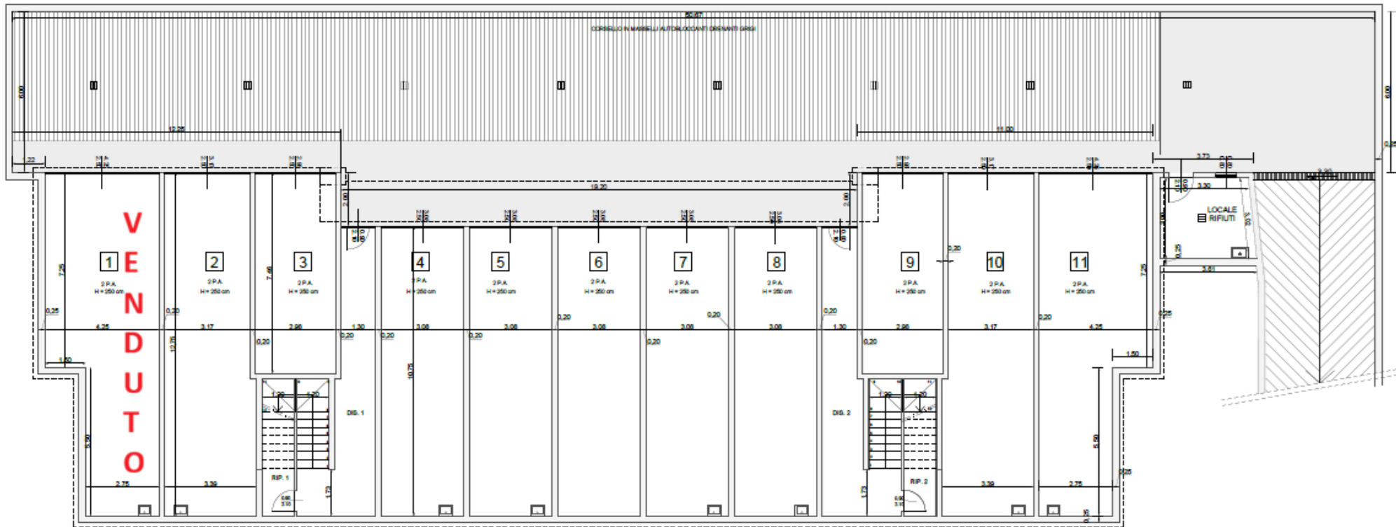
PIANTA PIANO INTERRATO
